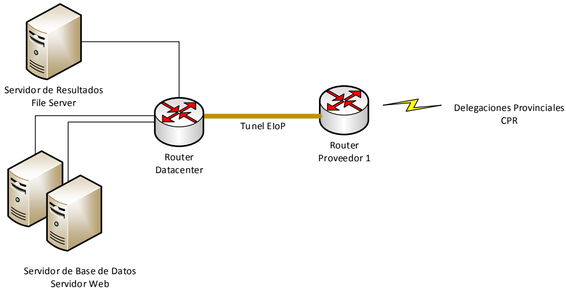
Figura 8. Procesamiento centralizado
